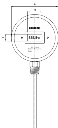
DI Bottom mount
